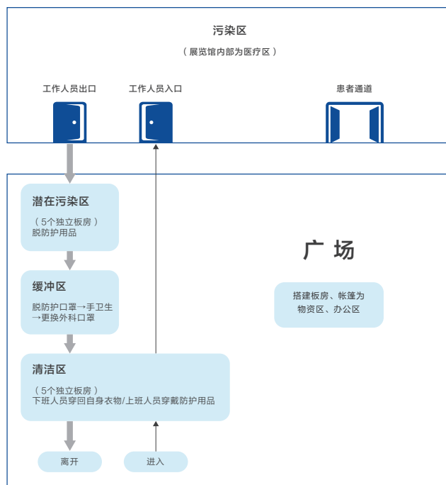
武汉某一家方舱医院（示意图）
